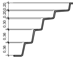
Detalhe 02
